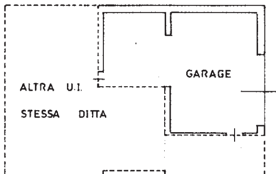
PIANTA PIANO INTERRATO H. = 235 ml
