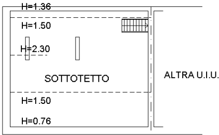
PIANO SOTTOTETTO
