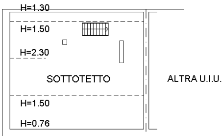
PIANO SOTTOTETTO
