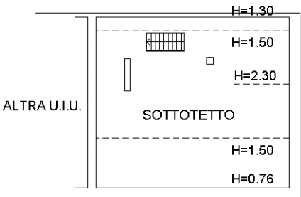
PIANO SOTTOTETTO
