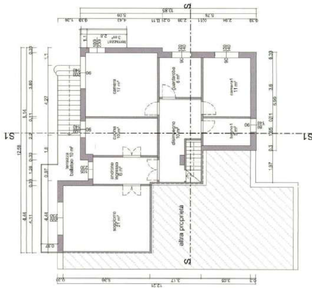
PIANTA PIANO PRIMO h ml.2.95 superficie utile netta mq.99 (Sc 91)
